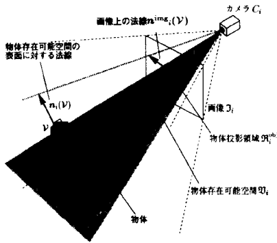
図4 画像上の法線と物体存在可能積空間の表面上の法線 Fig.4 A planar normal on image plane and a spatial normal on the surface of existence shadow space.
