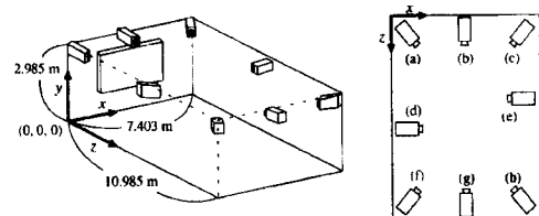
図 5 カメラレイアウト
